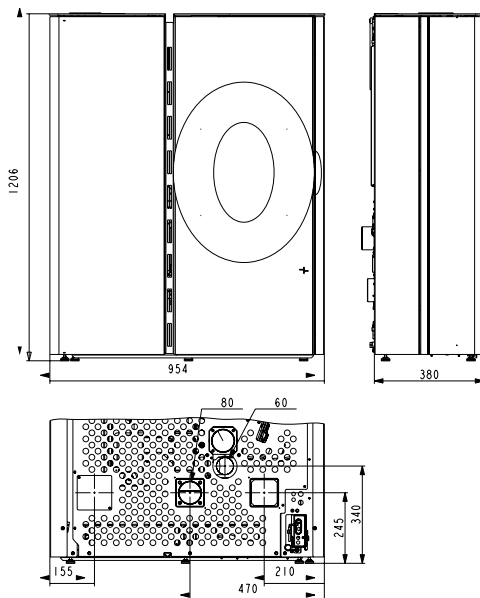
HSP 4.0-F2-03 TÜR OVAL Tür oval perl-grau, KV inkl. 2R Anschluss hinten li/re/mi 05 456 08 92 0000 EAN 90 027 42 48 0011
