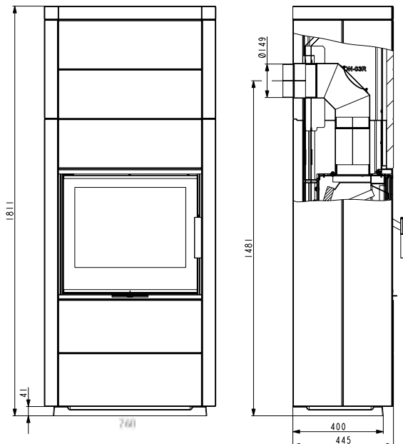
LEVI EASY Design „horizontal“, farblich individuell gestaltbar mit Spezialbeton, Einsatz: LEVI Easy 06 018 80 11 0000 EAN 90 027 42 46 5292
