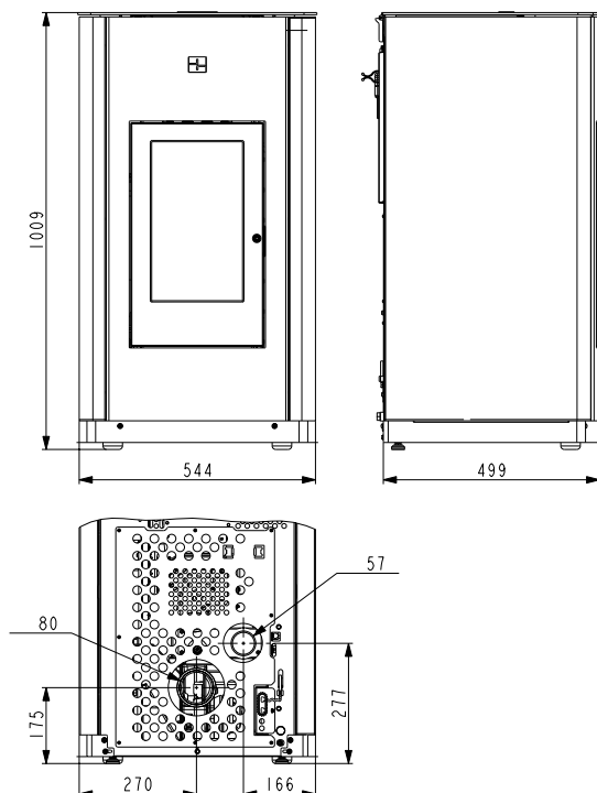
HSP 6 PELLETTO-IV perl-grau, perl-anthrazit 05 419 08 17 0000 EAN 90 027 42 46 0754
