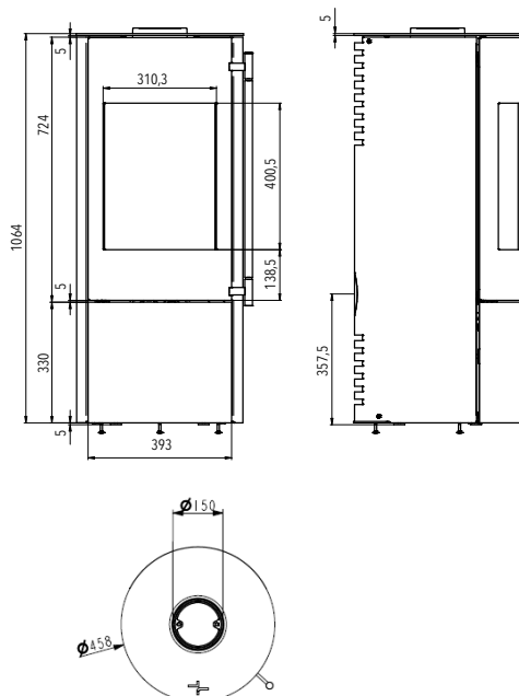
LURE MIT TOPPLATTE Speckstein für LURE und LURE HSC* Gewicht: 27 kg
