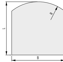
GLASPLATTE MIT SEGMENTBOGEN 1000 x 1000 / R = 800 mm 11 159 10 30 0000 EAN 90 027 42 39 2369
